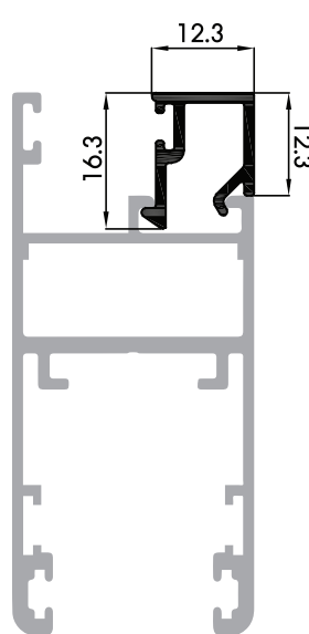
P-134573 กรอบบานมัลติล็อก ER ร่องสลักหลอดฐาน 5x5 มม. ยางอัด-ยางวางกระจก
