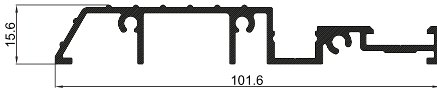
P-003603 เฟรมล่างประตูบานเปิด
