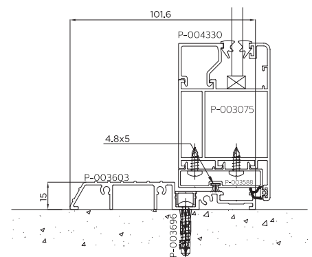
เฟรมล่างประตู ภายใน 4"
