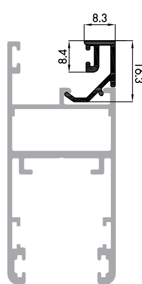
P-007227 ซีเสริมบาน ER
