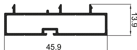
P-003588 ฝาตบกรอบบาน ด้านล่าง ร่องลึกหลอดฐาน 4.8x5 มม.
