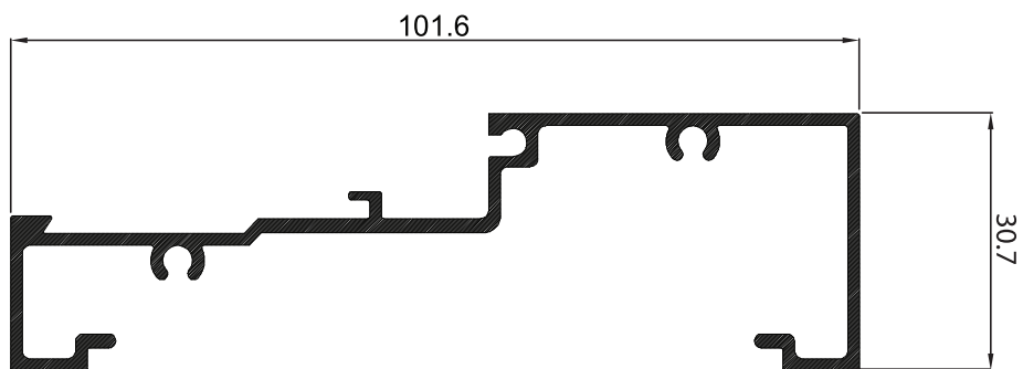
P-158432 กล่องเปิด
