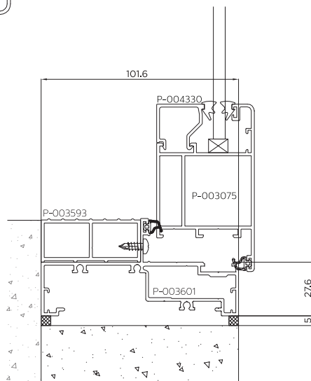
เฟรมล่างประตู ขนาด 4"
