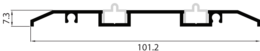
NEW P-154310 เฟรมล่างภายใน 2 ราง
