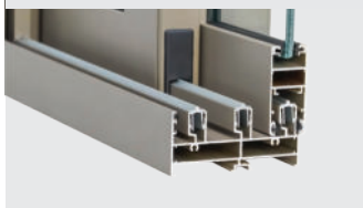
เฟรม 3 ราง ขนาด 4"
