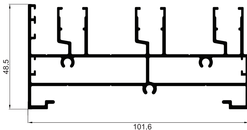
NEW P-124562 / 154307 เฟรมบานเลื่อน 4" ( 3 ราง ) ร่องลึกมาตรฐาน 5x5 มม.
