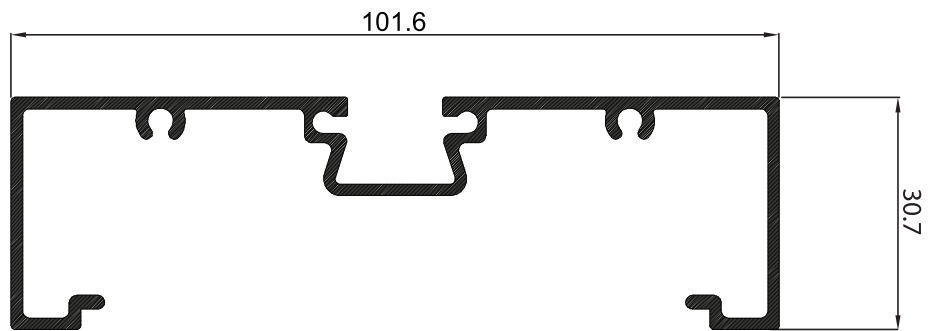
P-158434 กล่องรื่อง
