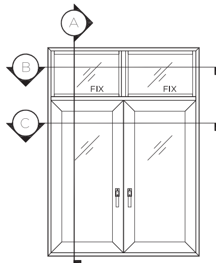
รายการเส้นบานเปิดคู่ ต่อช่องแสง
