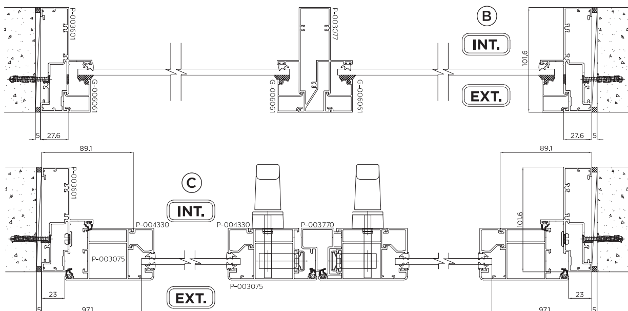
เฟรมบน-ล่าง หน้าต่าง ขนาด 4"
