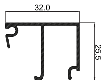
G-006061 คิ้วเหลี่ยม ER
