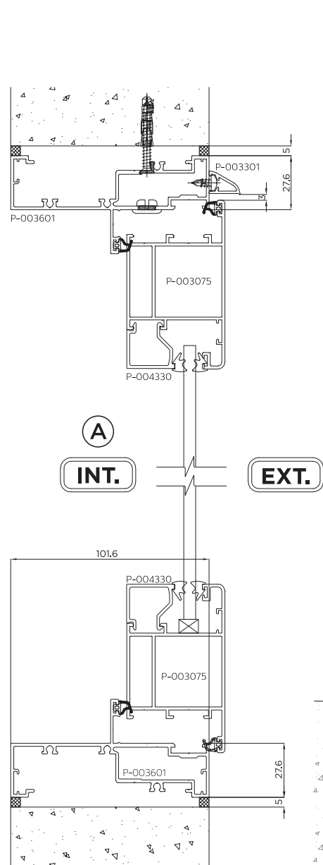
เฟรมบน-ล่าง หน้าต่าง ขนาด 4"
