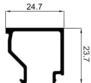
NEW P-004330 คิ้วเหลี่ยมบานเปิด ER 4"
