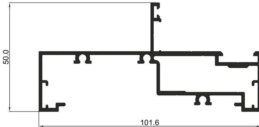
P-003601 เฟรมบานเปิด ยางลูกโป่งฐาน 4.8x6.5 มม.
