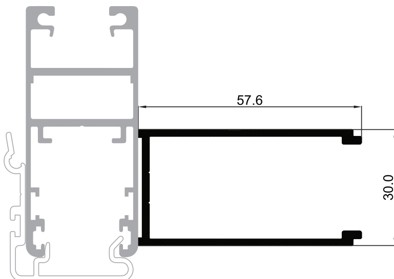
P-003000 เสาเสริมความแข็งแรง
