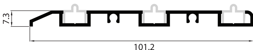
NEW P-154309 เฟรมล่างภายใน 3 ราง
