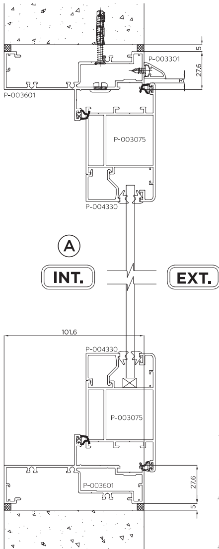
เฟรมบน-ล่าง หน้าต่าง ขนาด 4"
