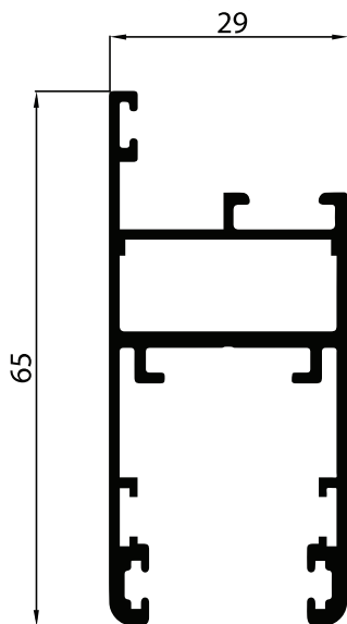
NEW P-154558 กรอบบาน ร่องสลักหลอดฐาน 5x5 มม. ยางยูกระจก 01,02
