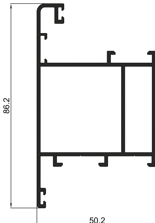
P-003075 กรอบบานเปิด ER 4" ยางลูกโป่งฐาน 4.8x6.5 มม. ยางอัด-ยางวางกระจก
