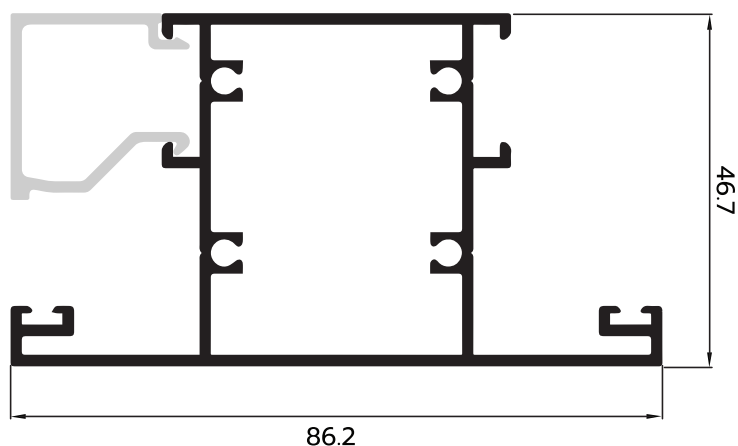
NEW P-154516 แบ่งกระจก 4" ยางอัด-ยางวางกระจก
