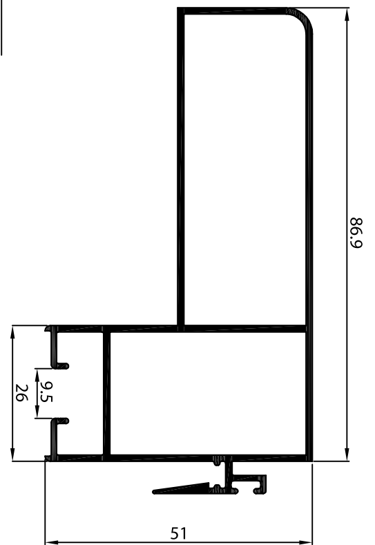
P-126783 เสาเกี้ยวหน้ากว้าง รับแรงลม 1.2 มม. ยางยูกระจก / สลักลาด 5x4
