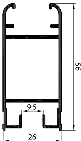
P-126780 เสากุกญแจ ล็อคหลายจุด Multi-point Lock ยางยูกระจก
