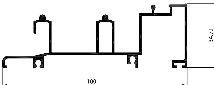
P-113512 เฟรม บน-ล่าง 10 ซม. (กรณีเตี้ย) ยางลูกโป่ง 4.7x6.5
