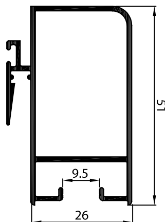
P-126781 เสาเกี้ยวหน้ากว้าง 1.2 มม. ยางยูกระจก / สลักลาด 5x4
