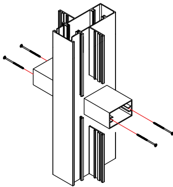
ภาพ Detail การเจาะและยึดของ แบ่งบานกับตัว P-123264 Adapter แบ่งบาน **กรณีไม่ใช่ สดดี ให้ใช้สกรูแบบเกลียวป้อย M4 แทน
