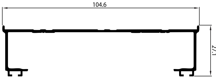
NEW P-154785 เฟรมข้าง ยางลูกโป่ง 4.7x6.5
