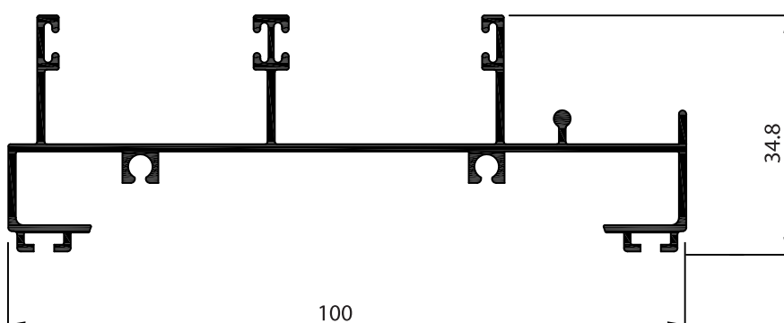
P-113508 เฟรมข้าง 10 ซม. ยางลูกโป่ง 4.7x6.5 / สลักตา 5x4
