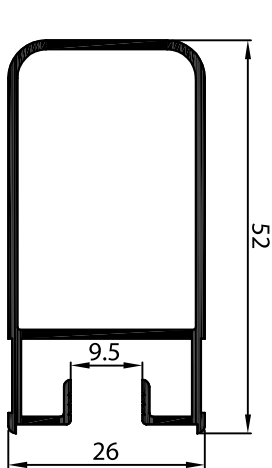
P-126779 เสากุกญแจ ล็อค 1 จุด Single Lock 1.2 มม. ยางยูกระจก
