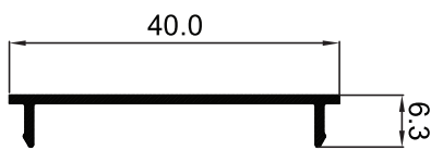
P-003400 ฝาแคป Capping
