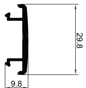
P-003042 ฝาปิดเสาเสริมความแข็งแรง
