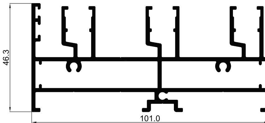
P-003584 เฟรมบานเลื่อน 4" ( 3 ราง )
