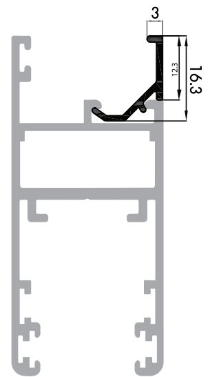
P-123119 คิ้ว (ระยะ 20 มม.)
