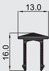
P-009511 រាងស្រោច ប្រភេទ-ស្រោច
