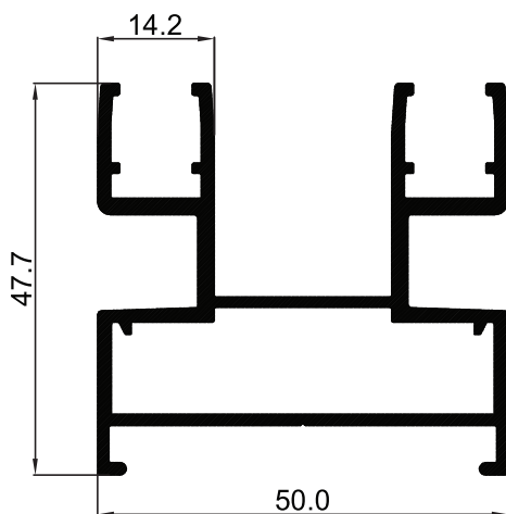
P-009519 ប្រភេទស្រោច 2 រាង
