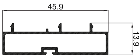
P-003588 ฝาตบกรอบบาน ด้านล่าง
