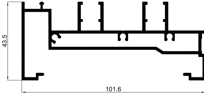
P-006970 เฟรมบน-ล่างบานเลื่อน 4" ( 2 ราง )
