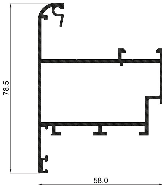
P-009517 กรอบบานหน้าต่าง ER
