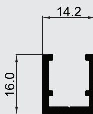
P-006968 ប្រភេទ ER
