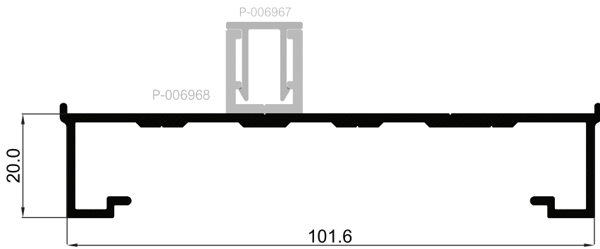
P-006969 เฟรมข้างบานเลื่อน 4"
