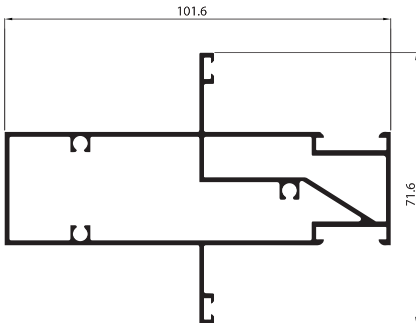
P-003077 แบ่งบาน
