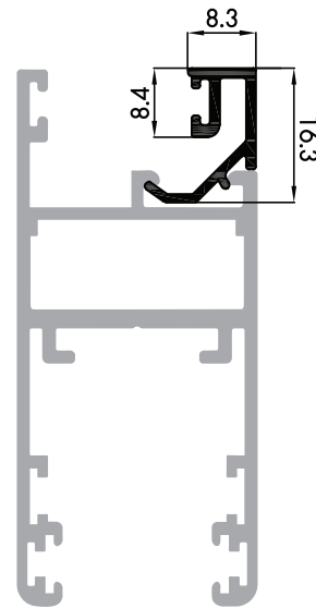
P-123118 คิ้ว (ระยะ 10 มม.)
