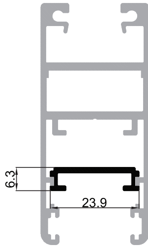
P-007227 ซีเสริมบาน ER
