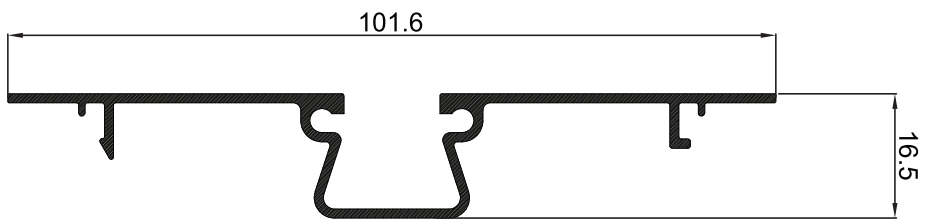
P-003093 ถาดร่องยาว ER
