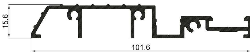
P-003603 เฟรมล่างประตูบานเปิด
