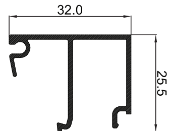
P-006061 คิ้วเหลี่ยม ER
