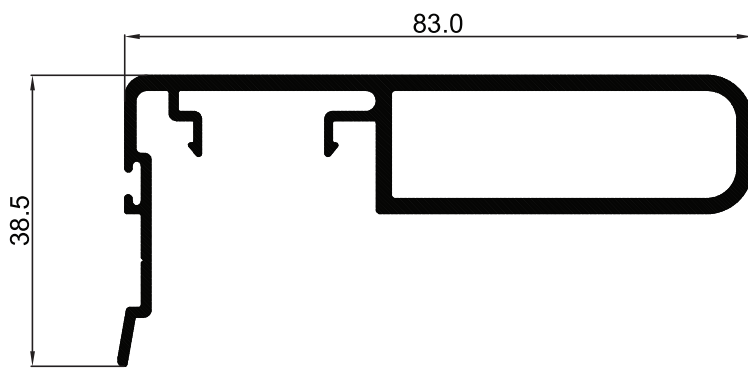
P-009514 ตบเสาตบเกี่ยวเล็ก ER
