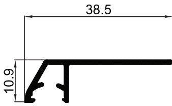
P-003594 Headsill ขยาย
