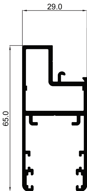
P-003590 กรอบบาน
